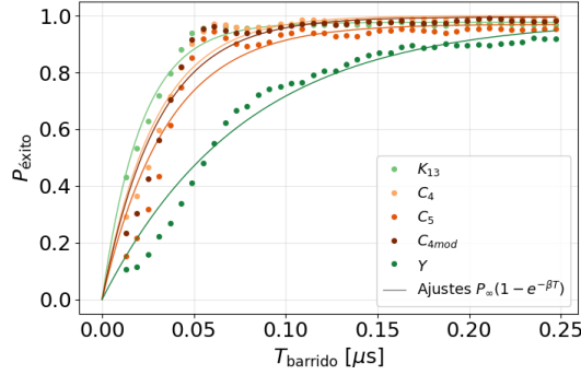
(c) Resto del catálogo, A = 50 \text{ rad}/\mu\text{s}
