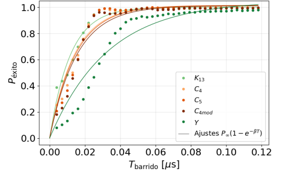
(d) Resto del catálogo, A = 100 \text{ rad}/\mu\text{s}
